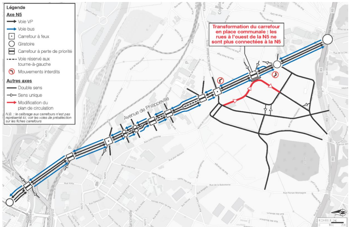
Figure 41 – Aménagements BHNS sur le secteur "Nord R3" (N5)
