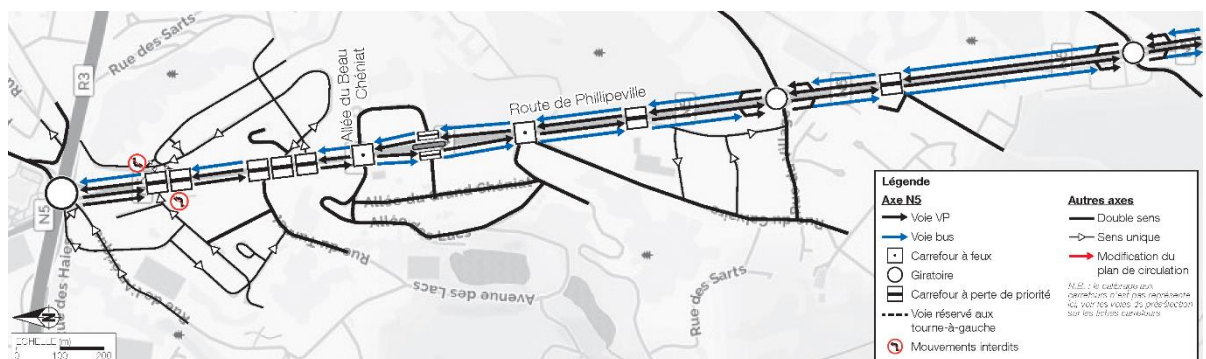
Figure 43 – Aménagements BHNS sur le secteur "Sud R3" (N5)
