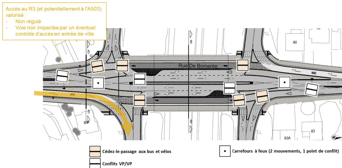
Figure 20 - Aménagement et gestion des conflits du carrefour N53/R3
