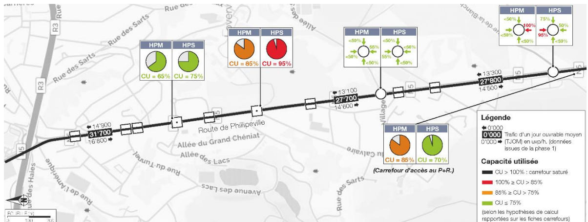
Figure 44 – Capacité utilisée des carrefours sur le secteur "Sud R3" (N5)
