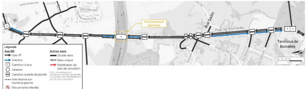
Figure 19 – Aménagements BHNS sur le secteur "Sud place" (N53)
