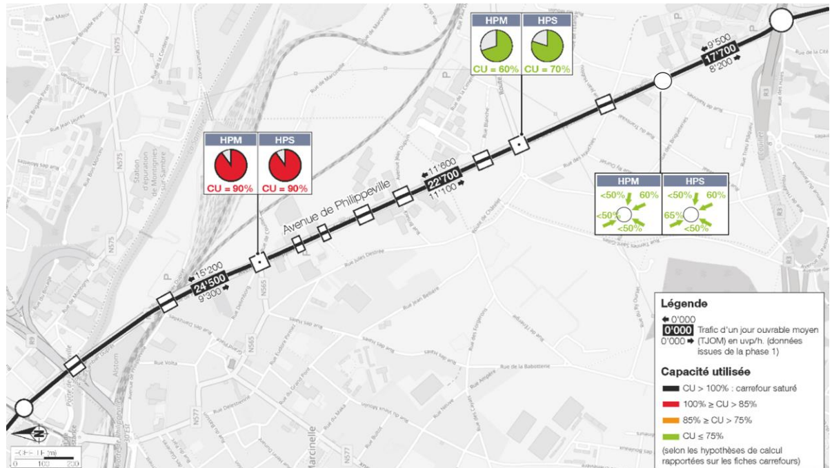
Figure 42 – Capacité utilisée des carrefours sur le secteur "Nord R3" (N5)
