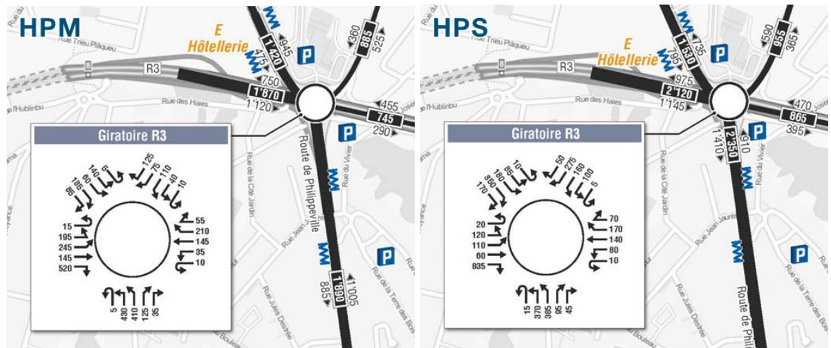
Figure 47 – Charges de trafic aux heures de pointe sur le giratoire "R3" (09. 2014)
